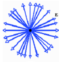
Onda natural
