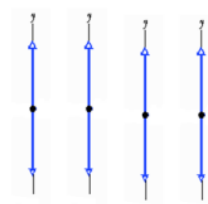
Onda planopolarizada
