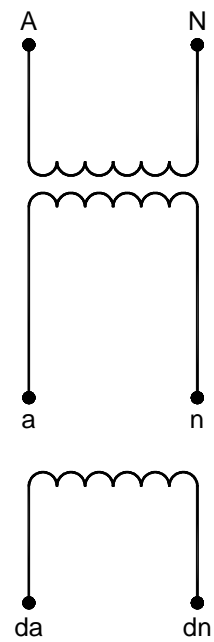
Figura 14. Transformador monofásico con devanado de tensión residual
