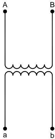
Figura 6. Transformador monofásico con terminales totalmente aisladas y un solo circuito secundario
