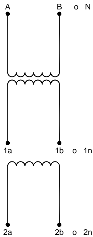
Figura 9. Conjunto monofásico con dos circuitos secundarios
