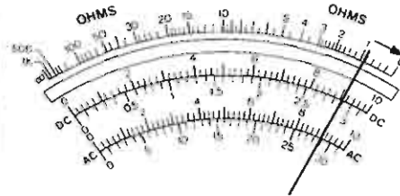
Selector de reglaje en R-1
