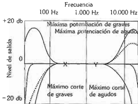
Efecto de los controles de graves y agudos Este gráfico muestra la alteración en los niveles de salida que se puede obtener con estos controles. La línea de puntos muestra el efecto de instalar un corte intermedio de graves y agudos.
