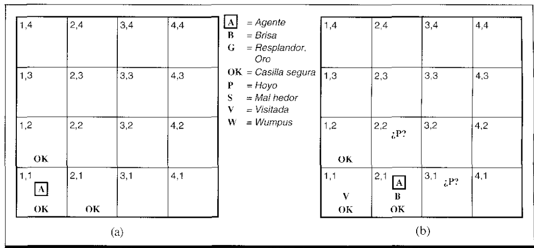
Figura 7.3 El primer paso dado por el agente en el mundo de wumpus . (a) La situación inicial, después de la percepción [ Nada, Nada, Nada, Nada, Nada ]. (b) Después del primer movimiento, con la percepción [ Nada, Brisa, Nada, Nada, Nada ].
