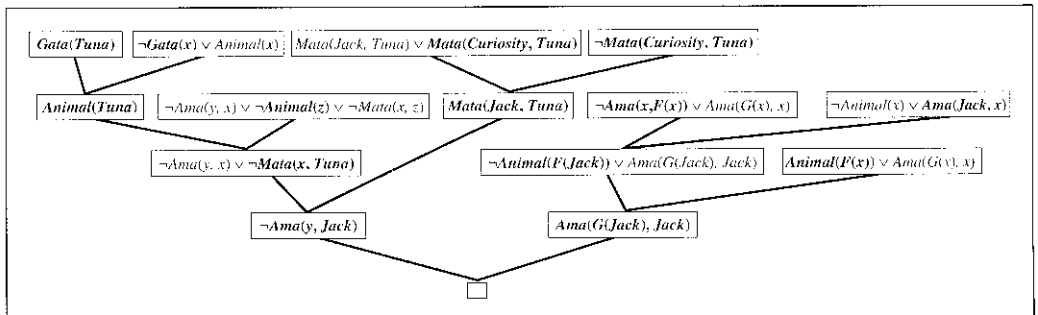
Figura 9.12 Una demostración mediante resolución de que Curiosity mató a la gata. Fíjese en el uso de la factorización en la derivación de la cláusula \text{Ama}(G(\text{Jack}), \text{Jack}) .
