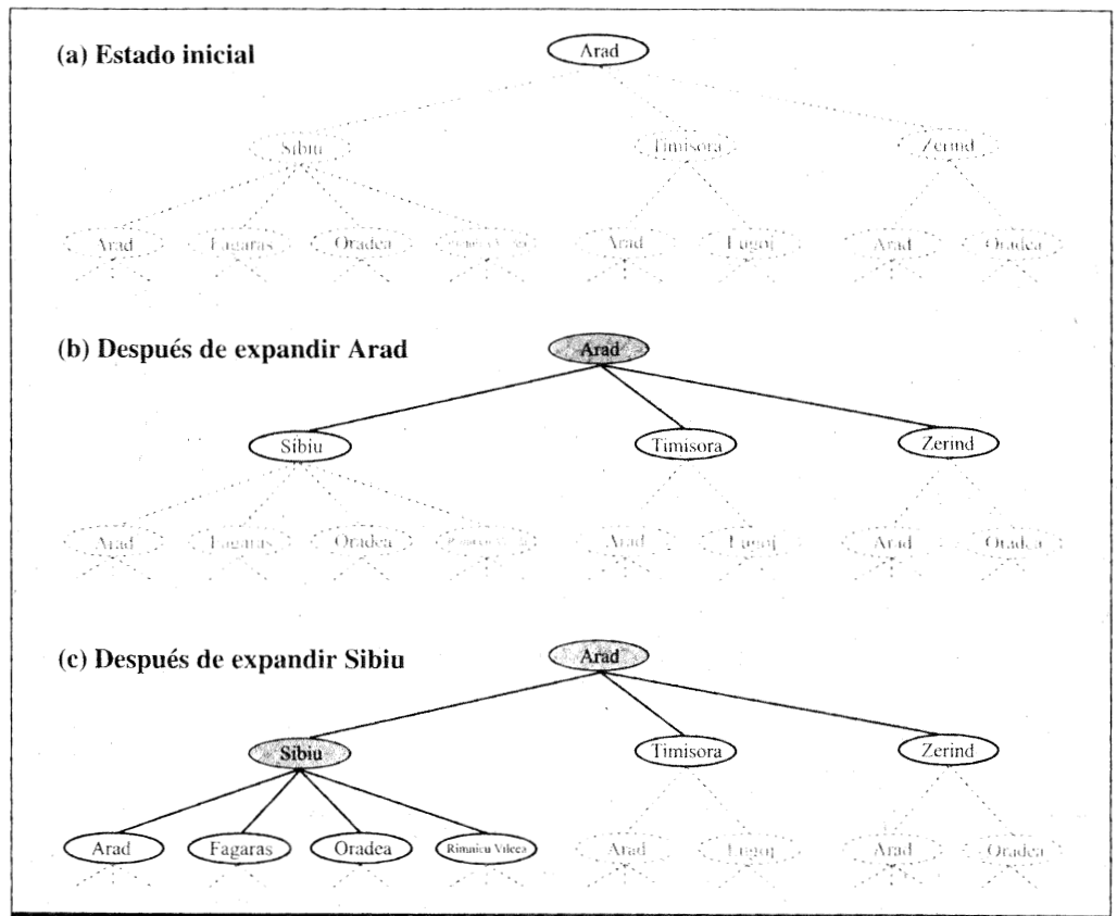
Figura 3.6 Árboles de búsqueda parciales para encontrar una ruta desde Arad hasta Bucarest. Se sombrea los nodos que se han expandido; los nodos que se han generado pero todavía no se han expandido se rodean en negrita; los nodos que todavía no se han generado se marcan con líneas discontinuas.
