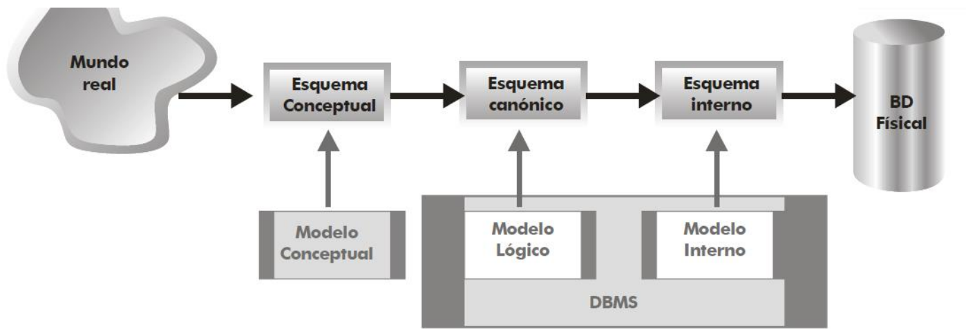
Ilustración 5, Clasificación de los modelos de datos
