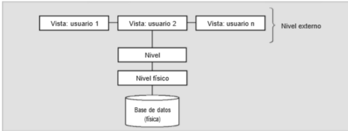
Fig. 1.2 Niveles de la base de datos.
